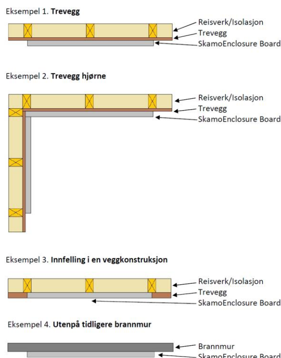
Fig.1 Montering av SkamoEnclosure Board som brannmur.
