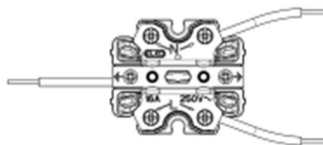
Koblingsskjema
