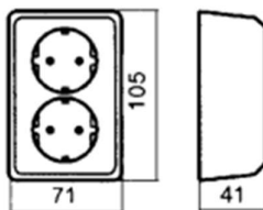
Målskisse
