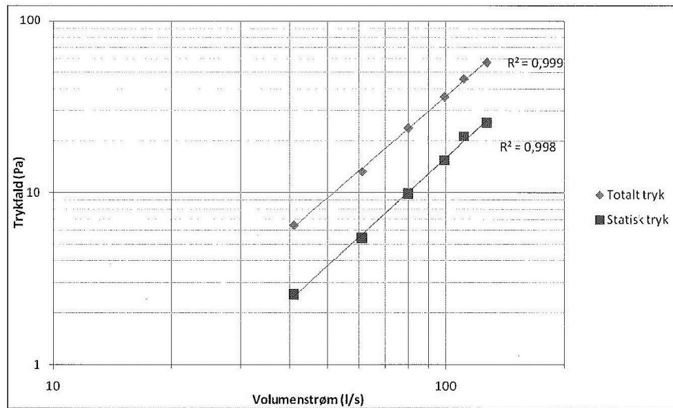
Kapacitetsdiagram: Stor hætte tilsluttet Ø160 mm rør.
