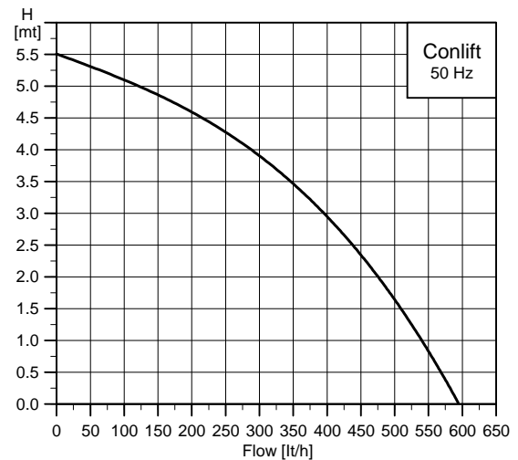
Fig. 20 Ydelseskurve
