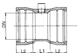
S-9171-4 Dobbelmuffe
