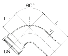
S-9674 Muffespiss bend 90°
