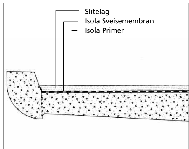
Fig 5. Føringskant brudekke
