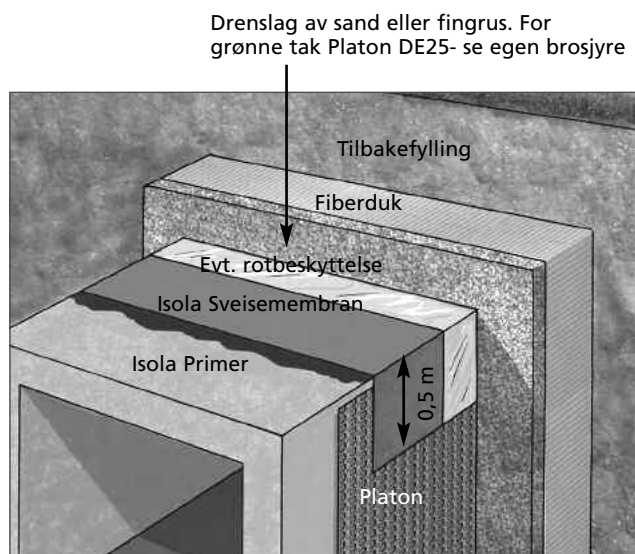
Fig. 2 Kulverter og tunneler med tilbakefylling
