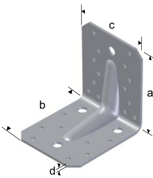
Type V4
