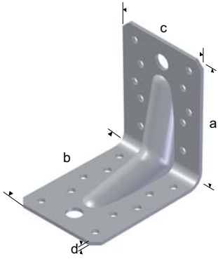
Type V1
