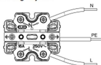
Koblingsskjema
