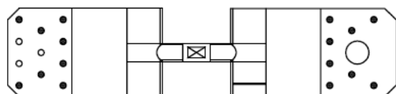
8 + 8 M5 Bolts
