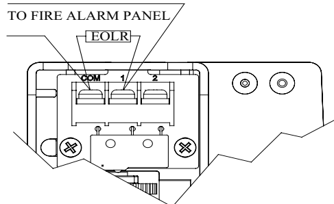
Anslutning av flödessignal Figur 5
