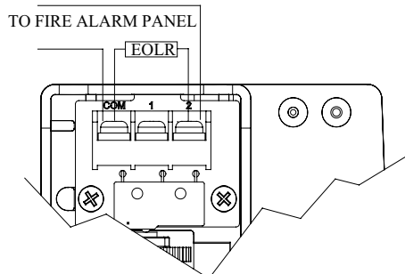
Signalanslutning vid lågt tryck Figur 4
