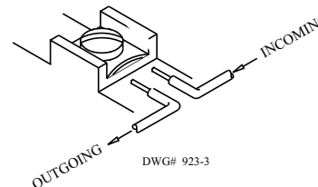
Anslutningsplint Figur 2
