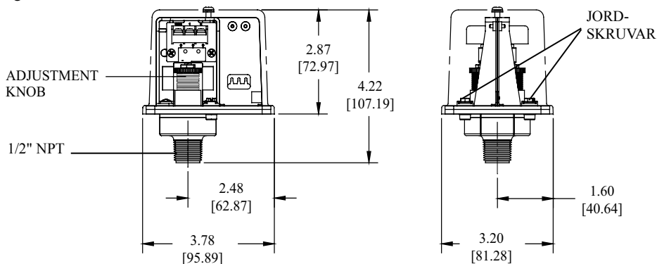
Mått Figur 1
