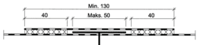
Fig. 54 c Feste av takfolie gjennom bane med overdekning
