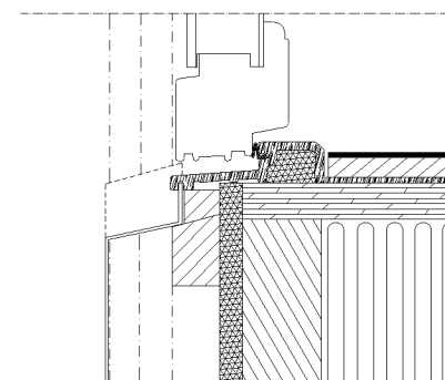
SNITT A-A
