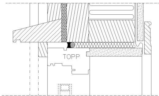
SNITT C-C
