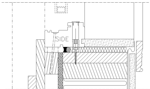
SNITT B-B
