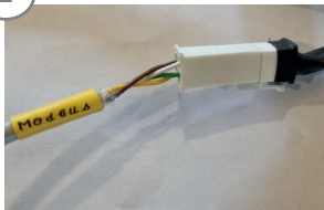
Kopplas till kabel märkt Modbus på toppen av aggregatet
