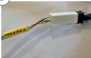
Kobles til kabel merket Modbus på toppen av enheten
