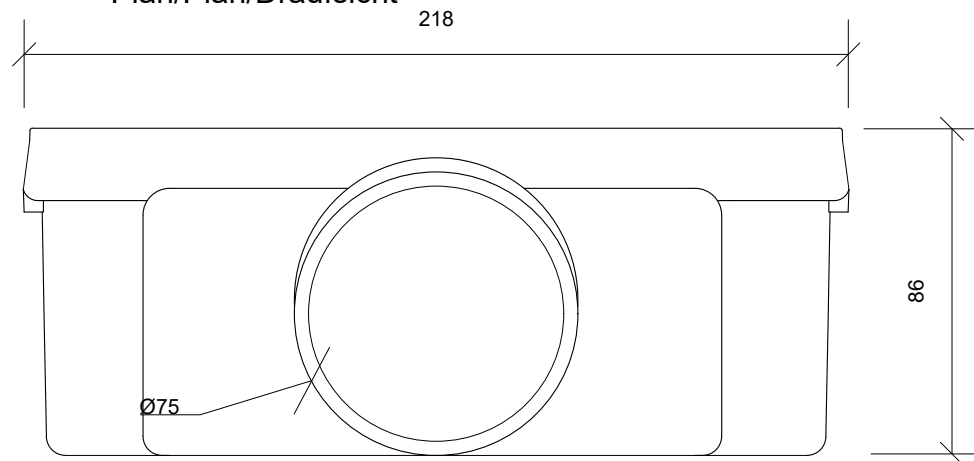
Plan/Plan/Draufsicht
