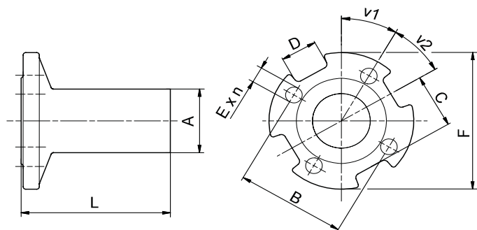
Fig. 22 Målskitse og billede af overgangsstykkerne gevind-til flange
