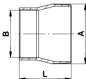
Fig. 23 Målskitse og billede af overgangsstykket gevind til gevind
