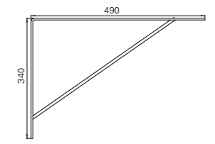
Konsoll SK 70
