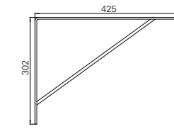
Konsoll SK 60
