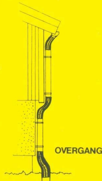
NEDLØP/OVERGANG FRA TAKRENNER
