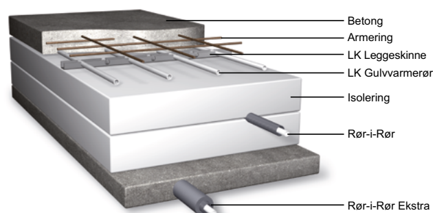
Forlegging av Rør-i-Rør i betongplate med gulvvarme.
