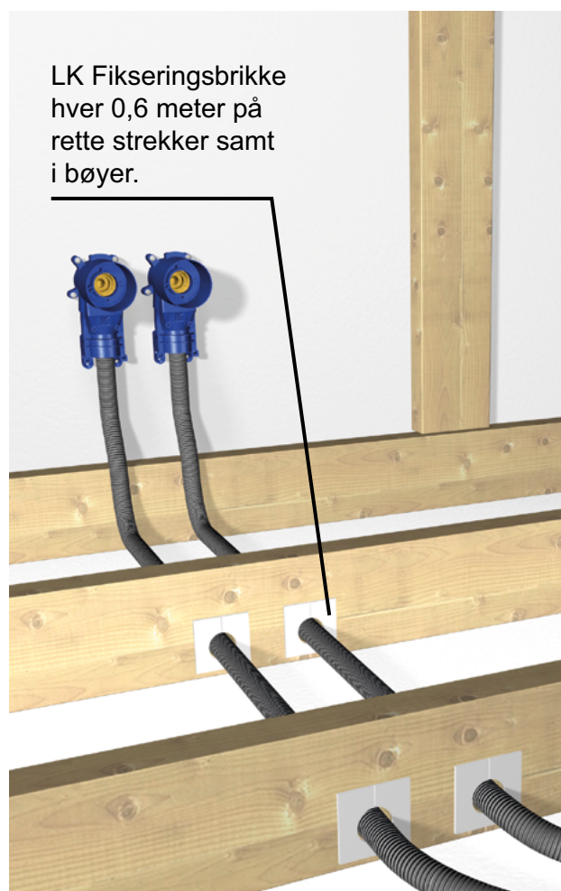
Fiksering av Rør-i-Rør i lektekonstruksjoner.
