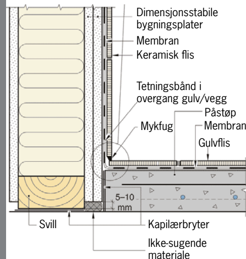
Prinsippskisse for overgang gulv/vegg (Tegningene er hentet fra Våtromsnormen)
