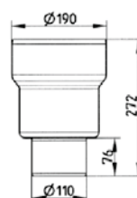
bunnutløp 3396325
