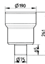
bunnutløp 3396324
