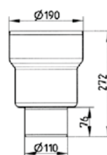
bunnutløp 3396325
