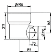
sideutløp 3396328
