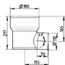
sideutløp 3396328
