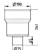
bunnutløp 3396324
