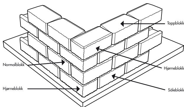
Bilde 7. Utvendig 90° hjørne.
