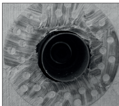
4. Smøremembran påføres inntil O-ring. Sjekk også at det ikke kommer smøremembran på boksforlenger!
