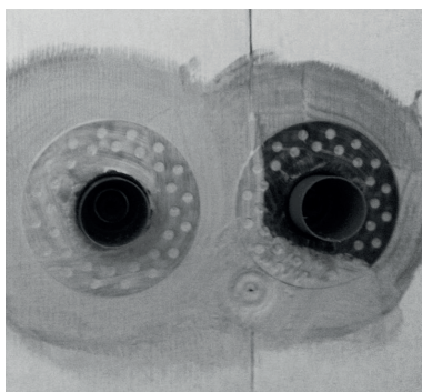
5. Legg et nytt lag smøremembran over mansjettene og ut på veggen.
