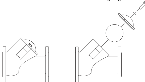
Fig. 37 Kontraventil
