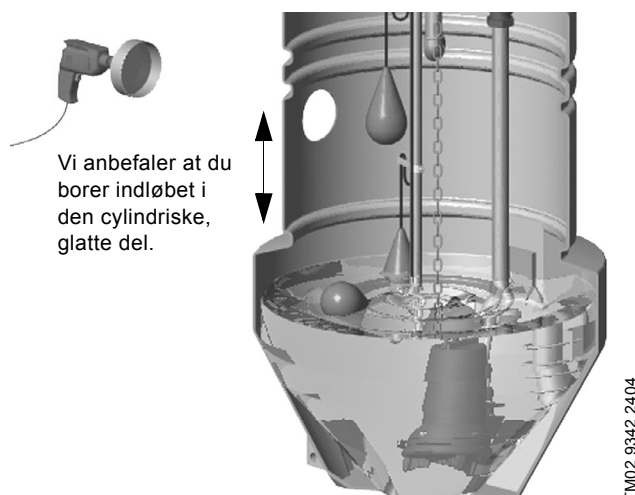
Fig. 21 Boring af indløb, Ø400-1000
