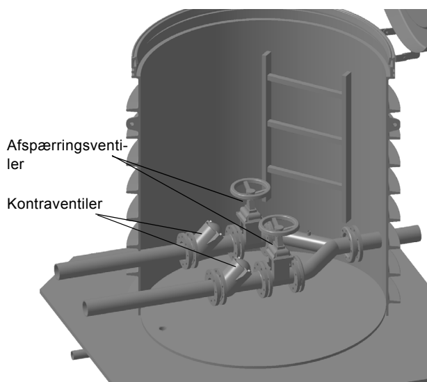
Fig. 20 Ventilkammer
