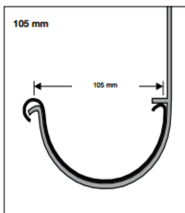
Figur 1 tverrsnitt av takrenne
