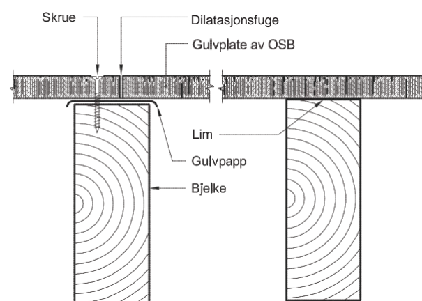
Fig. 5 Eksempel på utførelse av bevegelersfuge
