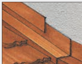
Overgangsbeslag mot mur
