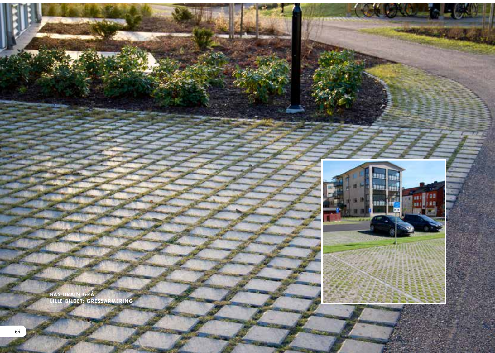
Bas Drain 210 x 210 x 100 mm med fas 22,7 stk/m 2 , ca 170 kg/m 2
