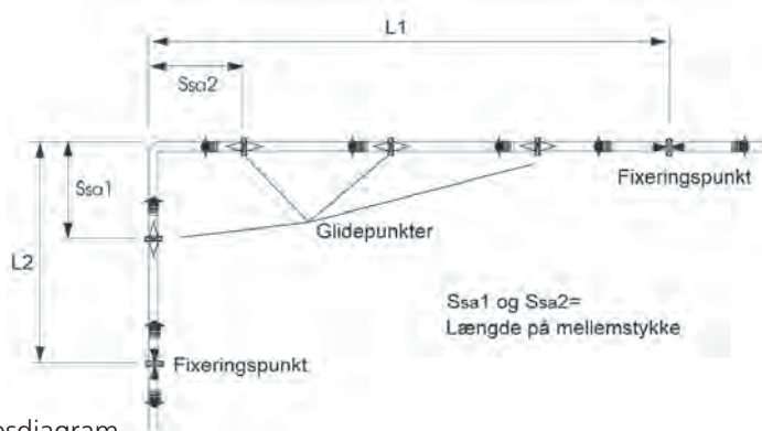
Varmeutvidelsesdiagram ( basert på \alpha = 0,025 \text{ mm} / (\text{m} \cdot \text{K}) )
