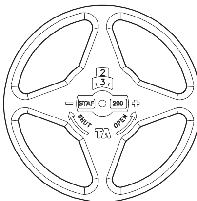
Fig. 2 Åpen 2,3 omdreininger
