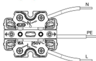
Koblings skjema
