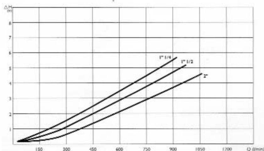
Trykktapsdiagram, vann ved 15°C
