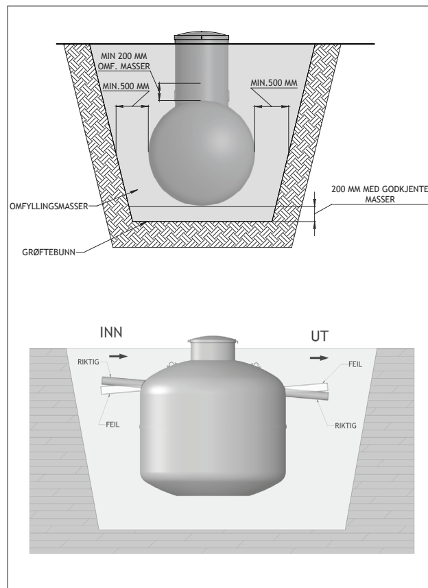
Figur 9: Standard installasjon
