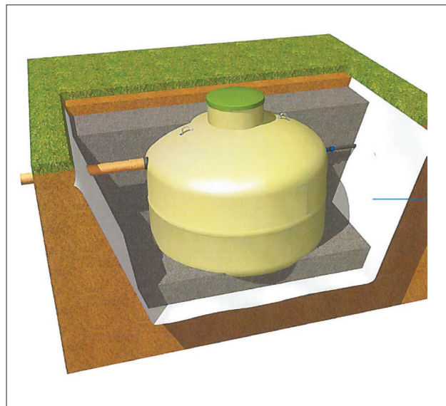
Figur 10: Grøftevegg sikres med fiberduk
