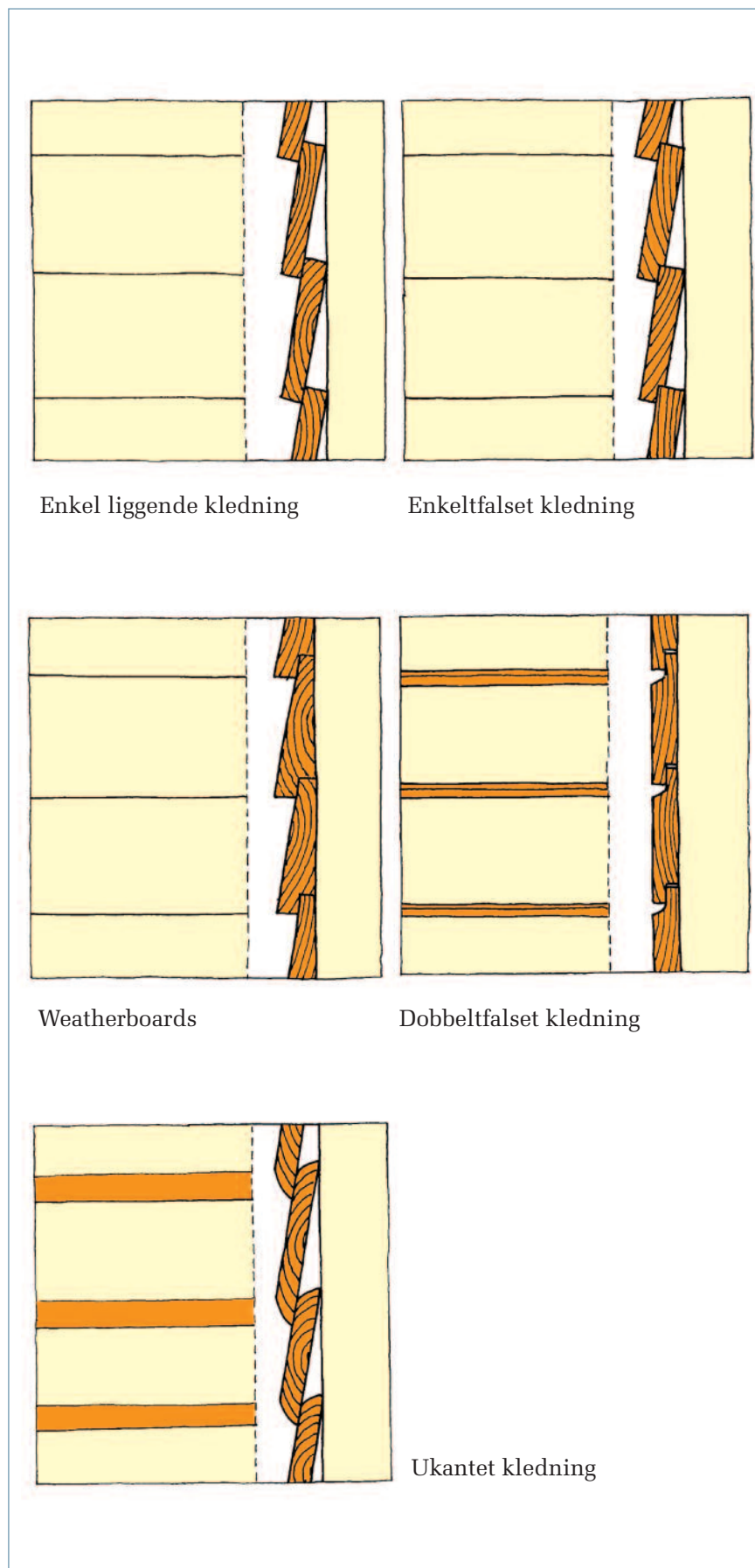
Figur 4. Eksempel på liggende kledning.
