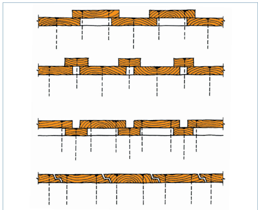
Figur 3. Riktig spikring av stående kledning.
