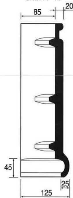
Snitt A - A
