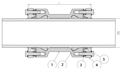
S-8160-1 Skjøtemuffe/Dobbeltmuffe for Drikkevann, vann og avløp
