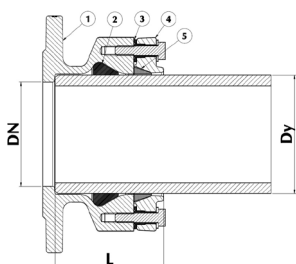
S-8160 Flensemuffe
