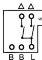
Koblingsskjema
