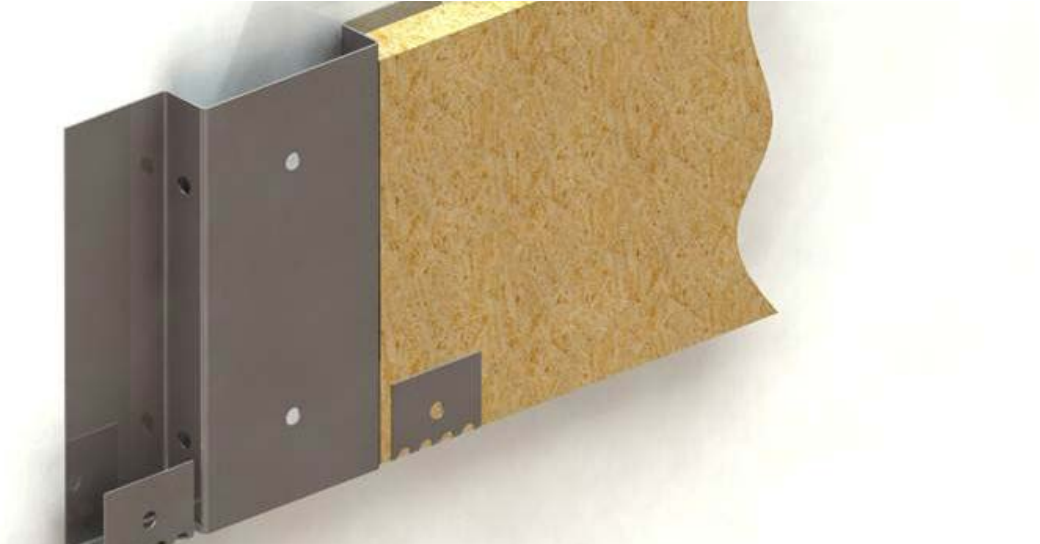
Monteringsbeslag for montering av spesialtilpasset OSB i format 2400X545 mellom stenderverk.
