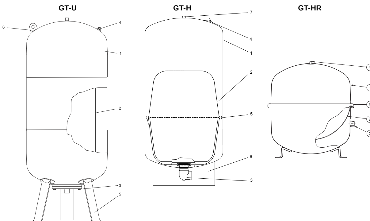
Fig. 1 Snittefigurer, eksempler på beholdere
