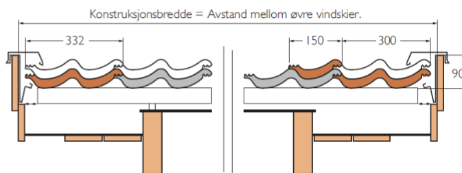
Konstruksjonsbredde uten bruk av gavstein
