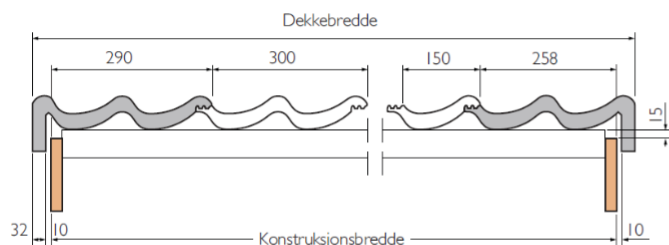
Konstruksjonsbredde ved bruk av gavstein
