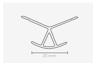
ALU PROFIL, 135° UTVEDIG HJØRNEPROFIL
