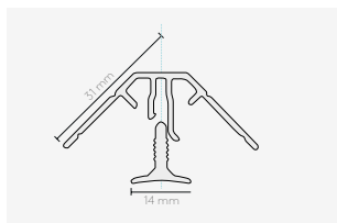
ALU PROFILER, TODELT INNVEDIG HJØRNEPROFIL
