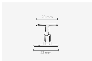
ALU PROFILER, TODELT SKJØTEPROFIL
