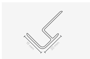
ALU PROFILER UTVEDIG HJØRNEPROFIL
