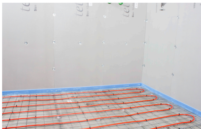
Benytt armeringsnett når dette er påkrevd.
