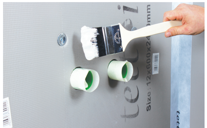
Påfør membran i et tilstrekkelig stort område.
