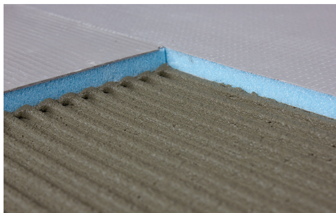
Platene legges med forskyvning.
