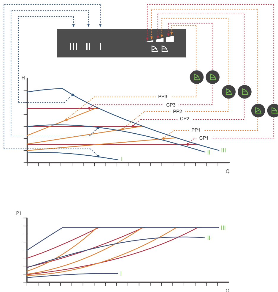
Fig. 25 Ytelseskurver i forhold til pumpens innstilling
