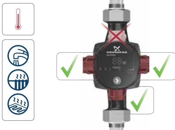
Fig. 3 Mulige posisjoner for kontrollboks, oppvarming og varmtvannssystemer
