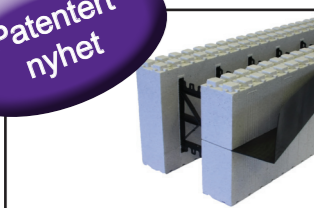
Thermomur 350 Radonblokk Med slisset spor for Radon vinkel. Finnes med åpen og tett ende og i Superblokk. Radon vinkel Til bruk sammen med Radonblokk. Skjøtes sammen med radonsperren.
