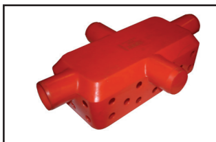
Jackon Radonbrønn Til oppsamling av radongass. 4 stk 110 mm uttak. Dekker ca 200 m 2
