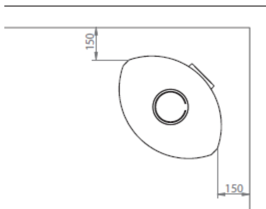
Afstand til brandbart med isoleret rørør
