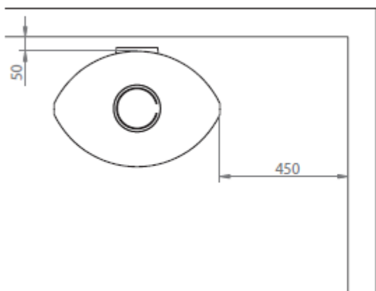
Afstand til brandbart med isoleret rørør
