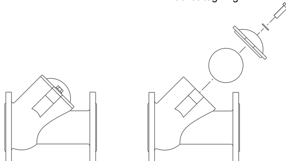
Fig. 37 Kontraventil
