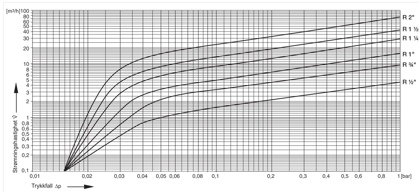
Fig. 1 Trykkfall inne i ventilen avhengig av vannmengden og tilkoblingsdimensjonen som er brukt
