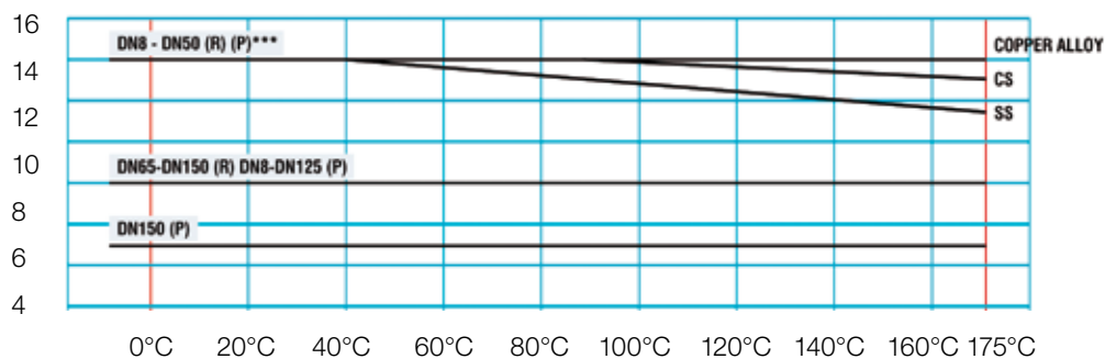
Förhållande temperatur / tryck i ventiltus
