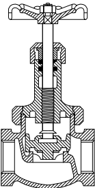
Kägelventil
