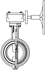
Vridspjällventil
