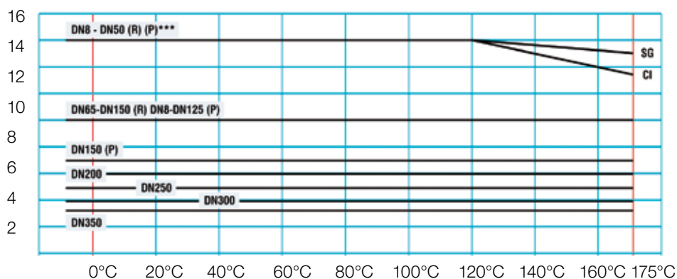
Förhållande temperatur / tryck i ventiltus
