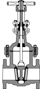
Slidventil
