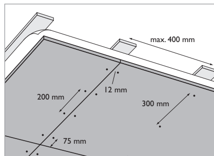
Etasjeskille tak
