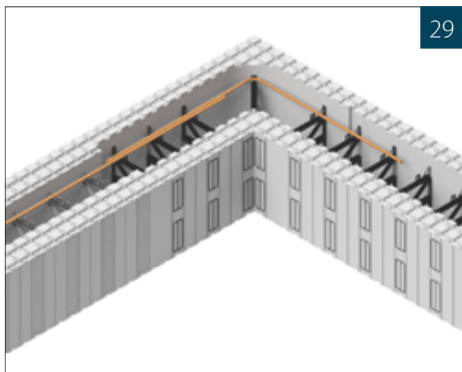
Fig. 29-30: Ved kombinasjon av Thermomur® 350 og 350HD i samme etasje (f.eks. der 350HD benyttes som bakvegg) bør området med overlapp mellom elementer ikke være større enn nødvendig. Man kan f.eks. bruke hjørneblokker i 350HD og vanlig 350-blokker i neste vegg.
