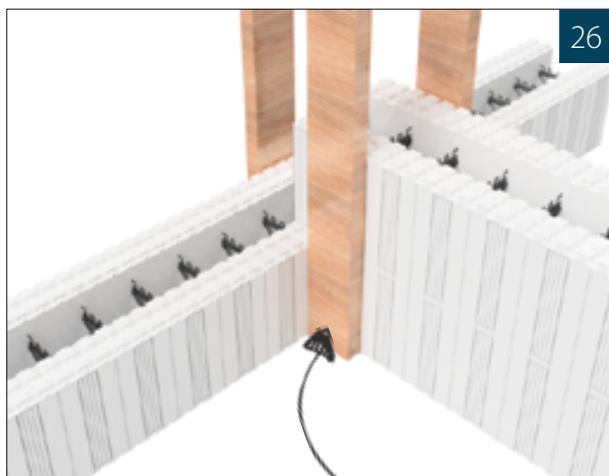
Trevirke 48 x 98 mm eller 22 x 98 mm justert forskaling
