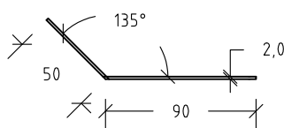
Snitt A-A
