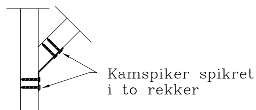
Snitt B-B
